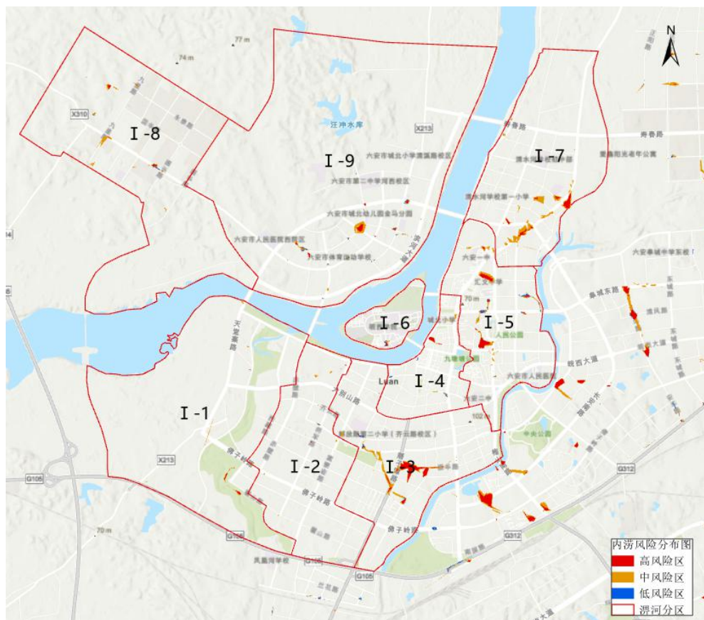
图 5.1- 6 淝河分区内涝积水风险图
