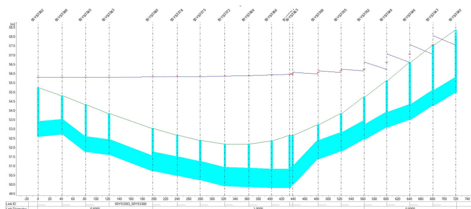
图 5.1- 27 长安南路管线纵断面图
