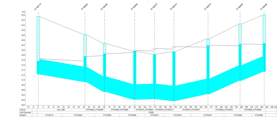
图 5.1- 11 民安巷管线纵断面
