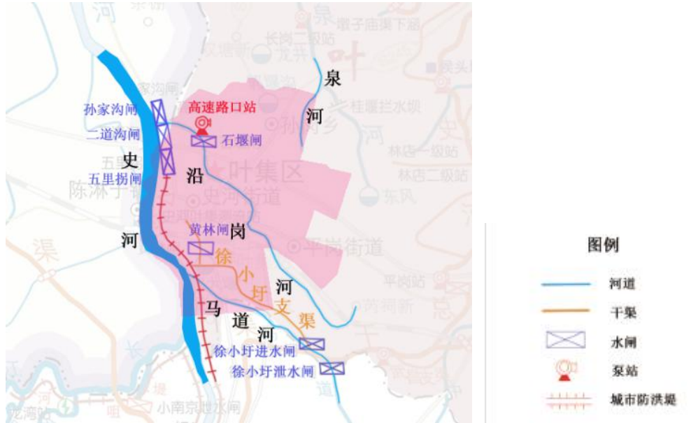
图 3.1- 2 六安市副城区防洪工程分布图
