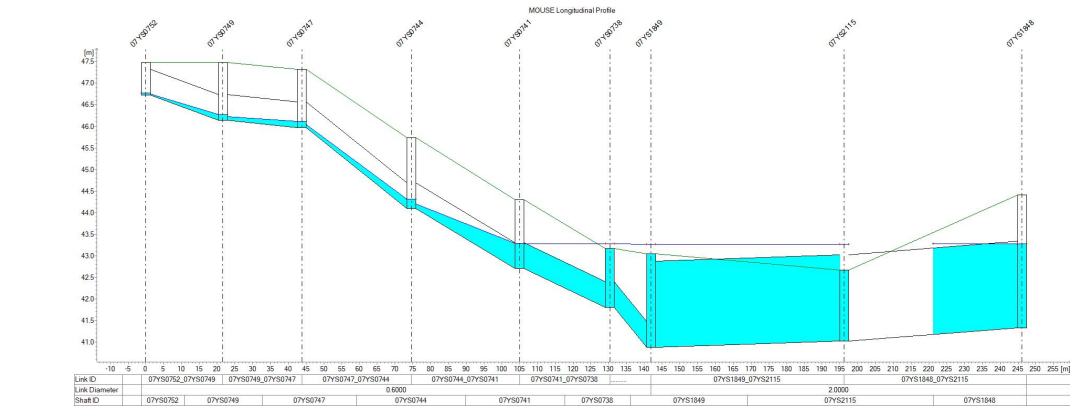
图 5.1- 8 文庙街排水（雨水）管网纵断面图
