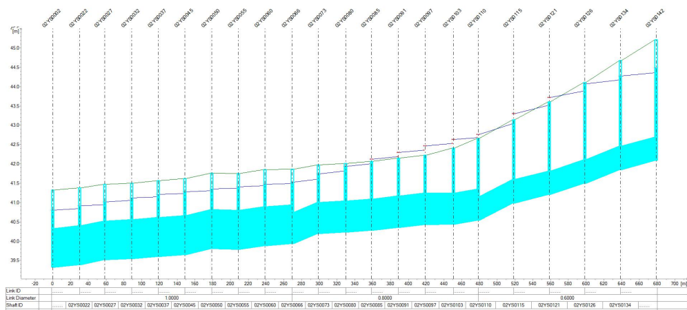
图 5.1- 52 二院门口管线纵断面图
