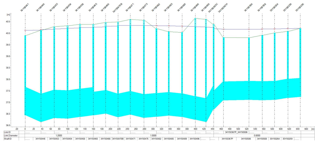
图 5.1- 48 正阳北路与蓼城路交叉口处管网纵断面
