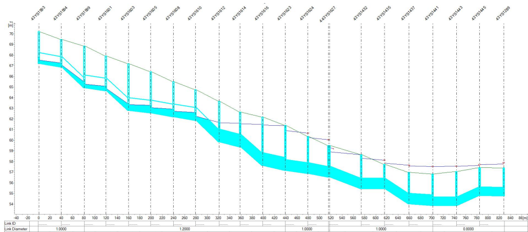
图 5.1- 22 安华路与皖西大道路口纵断面
