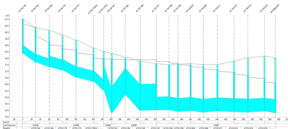
图 5.1- 25 晋善路纵断面
